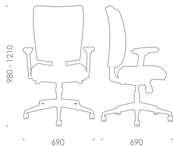
_BAS02 _Base alumínio polido 690 mm / 690 mm Polished aluminium base.
